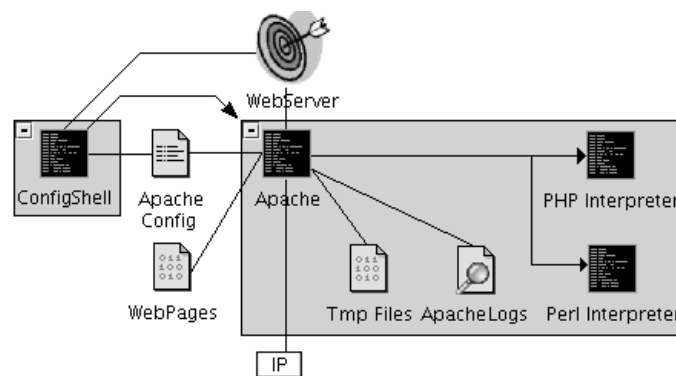
Figura 4. Visão expandida dos processos ConfigShell e Apache .
