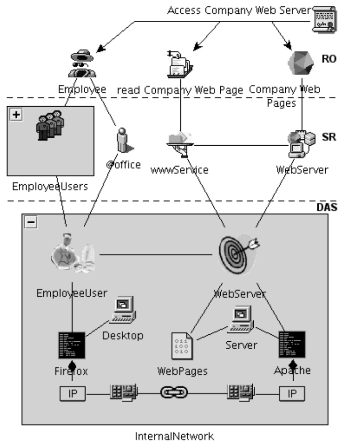
Figura 2. Modelo exemplo da política “Funcionários podem acessar o servidor web da empresa” utilizando MBM. Cada nível (RO, SR e DAS) é separado por uma linha tracejada
