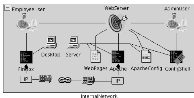
Figura 3. Nível DAS da política exemplo.
